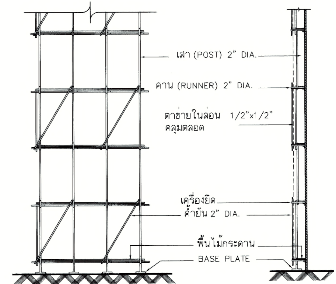
แบบขยายโครงเหล็กขึงฟ้าใบ
