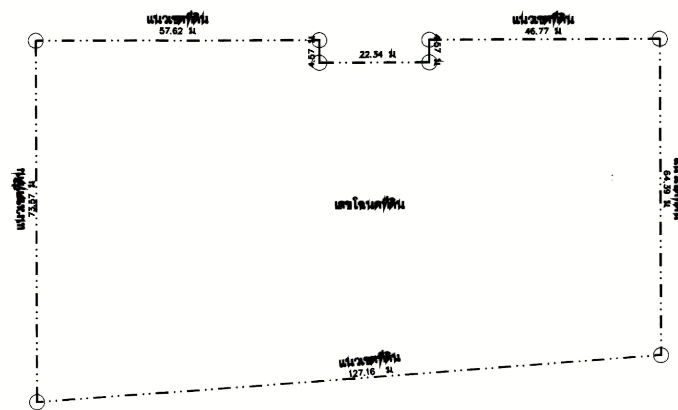
ผังโฉนดที่ดิน มาตราส่วน 1 : 200
